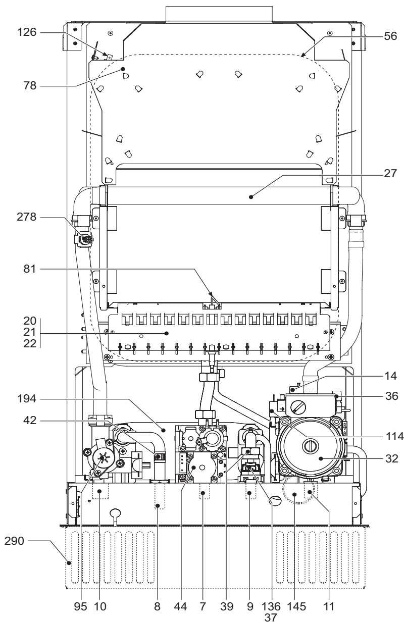
fig. 25 - Vista generale
