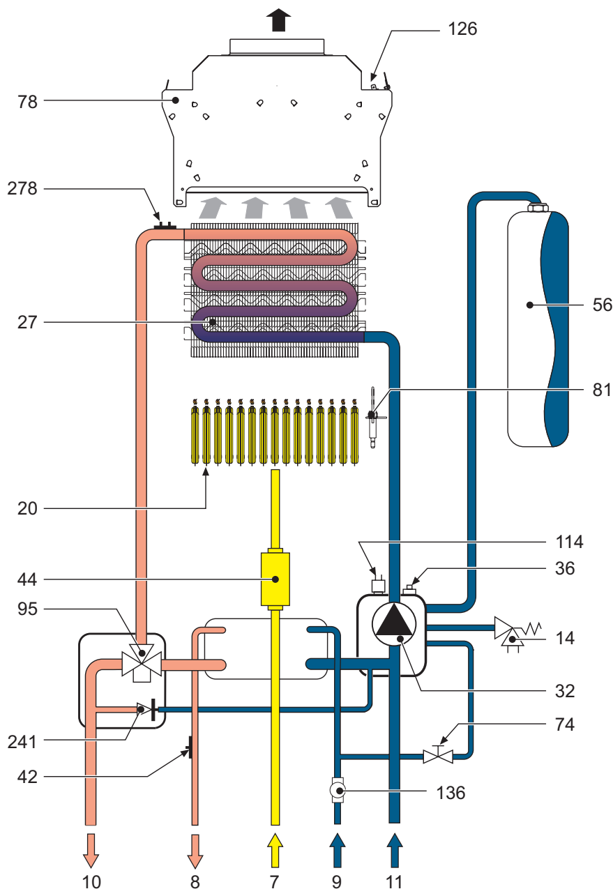
fig. 26 - Circuito idraulico
